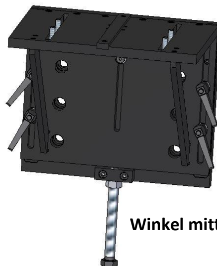
Messrad Anbauteile
